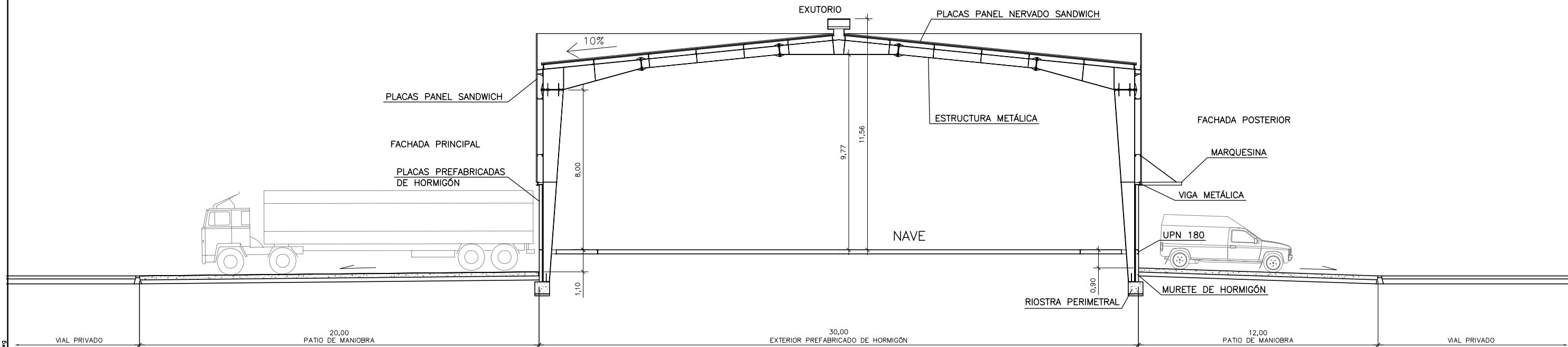
SECCIÓN A-A'
